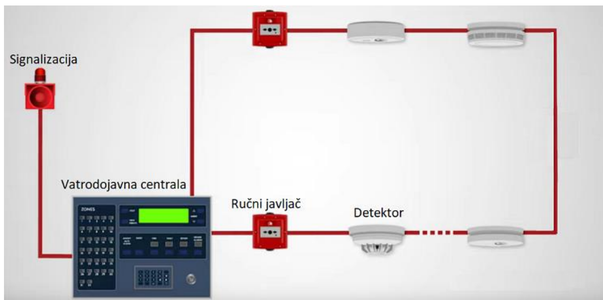
Slika 8. Princip postavljanja broskog vatrodojavnog sustava
