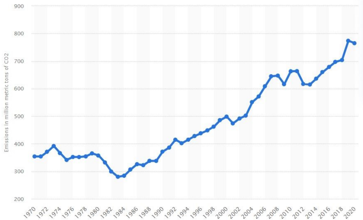
Grafikon 1 Emisije ugljičnog dioksida iz međunarodnog brodskog prometa diljem svijeta od 1970. do 2020. (u milijunima metričkih tona)
