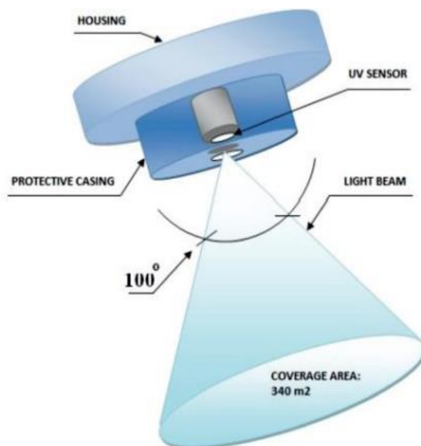
Slika 21 Ultraljubičasti detektor plamena
