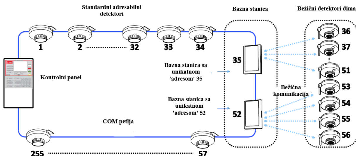
Slika 4 Primjer bežičnog vatrodjavnog sustava
