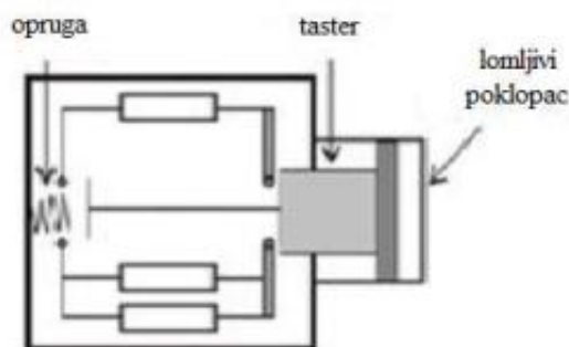
Slika 24 Građa ručnog javljača
