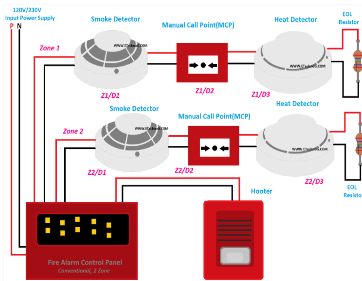
Slika 2 Konvencionalni vatrodojavni sustav
