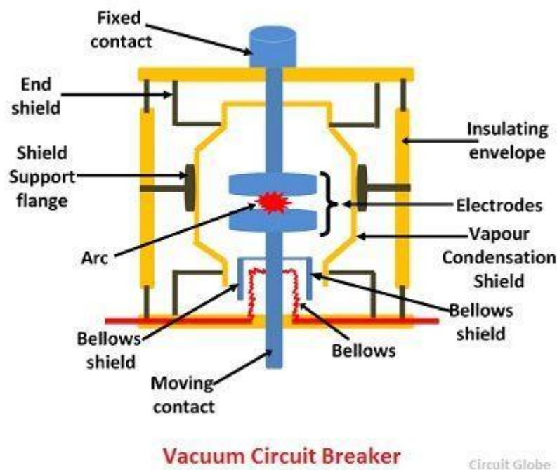
Slika 7-Vakumski prekidač
