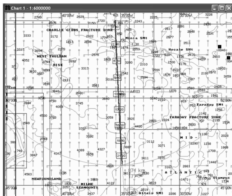
Slika 18 - Kretanje uljne mrlje prilikom djelovanja sile morske struje 10m/s i djelovanja vjetera 10 m/s
