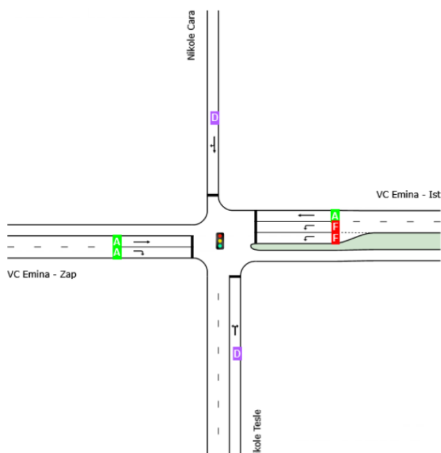
Slika 8. Prikaz stupnja uslužnosti za svaku pojedinu kretnju na raskrižju R39
