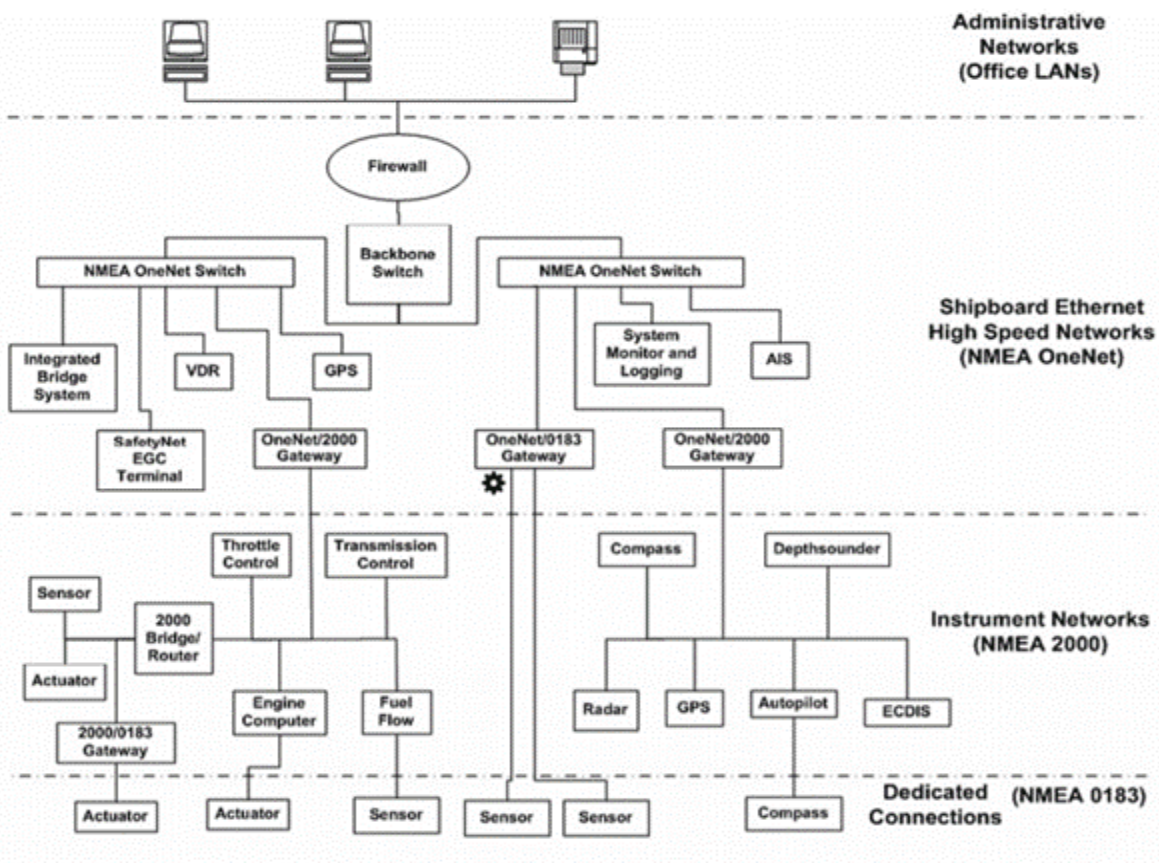
Slika 34. OneNet komunikacijska mreža na brodu, diagram povezivanja
