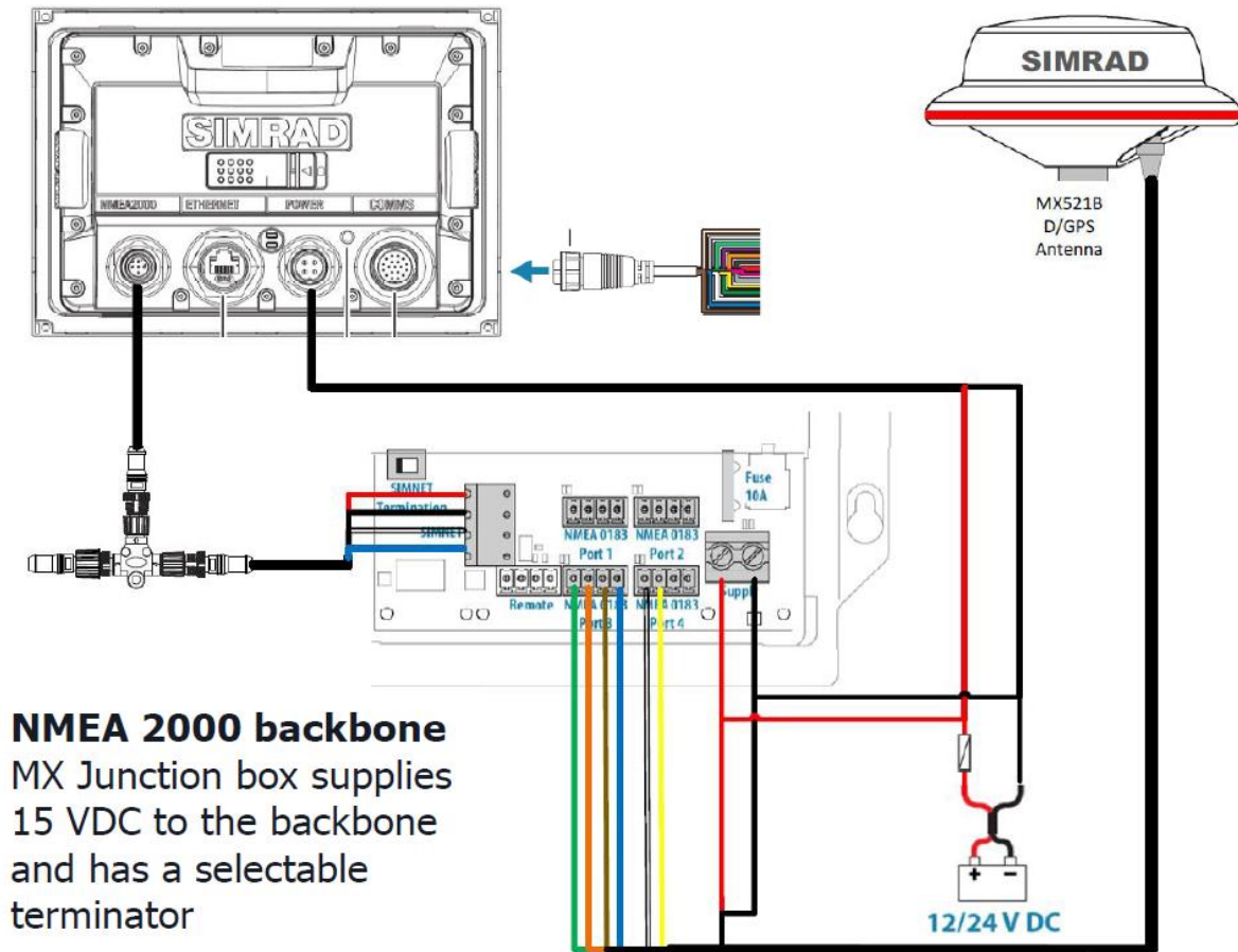
Slika 24. DGPS sustav MX 512 Simrad
