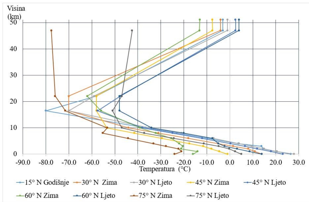
Slika 3.4.: Struktura temperaturnih profila troposfere po modelu standardne atmosfere USSAS 66
