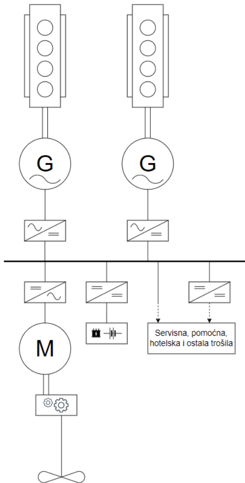
Slika 13: Topologija elektroenergetskog sustava broda s električnim sustavom propulzije i baterijskim skladištem energije (istosmjerna sabirnica) Izvor: Adaptirano iz: [79]
