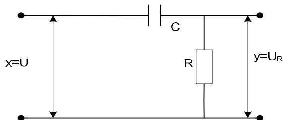
Slika 23. D član sa CR elementima
