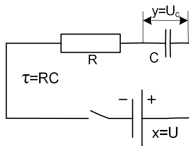
Slika 15. P_1 član sa RC elementima
