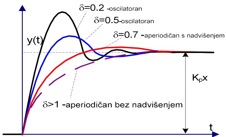
Odziv na odskočnu ulaznu pobudu
