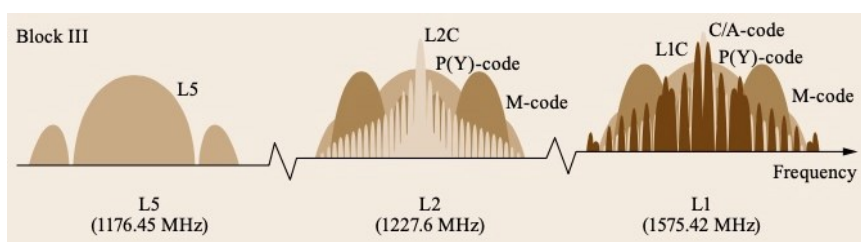
Slika 20. Prikaz GPS signala odašiljanih na pripadajućim frekvencijama
