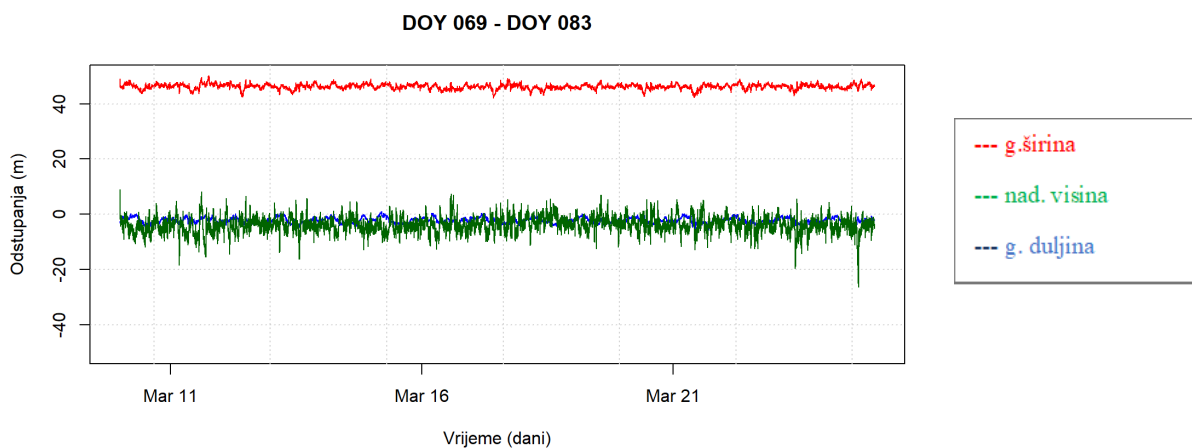
Slika 41. Modelirane vrijednosti odstupanja položaja za period od 10. do 24. ožujka 2015. (NYAL)
