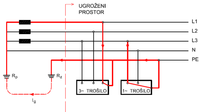
Slika 14. TT
