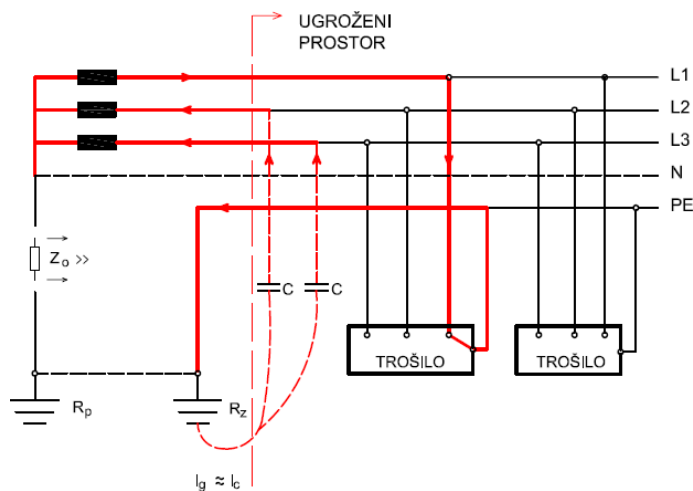
Slika 15. IT
