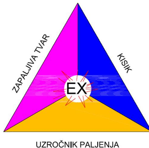
Slika 2. Trokut paljenja
