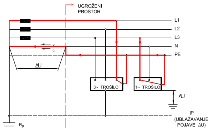
Slika 13. TN-C/S
