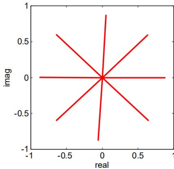
Slika 11. Niskopropusni ekvivalentni signali na kompleksnoj ravnini (jedna grupa)
