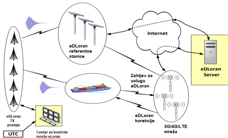
Slika 18. Koncept e-DLoran sustava
