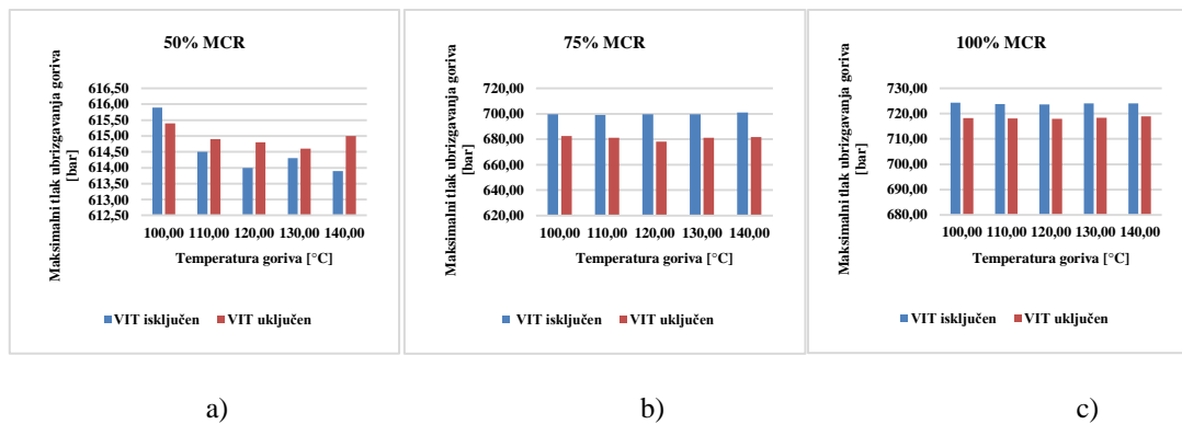
Slika 14. a), b) i c). Prikaz utjecaja VIT-a i temperature goriva na maksimalni tlak ubrizgavanja goriva pri razliitim optereenjim glavnog motora
