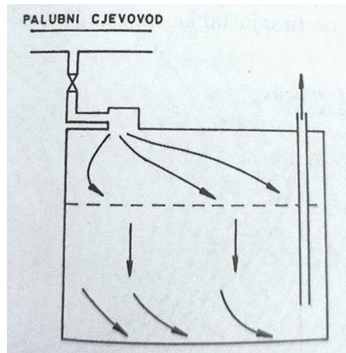
Slika 11 Inertiranje potiskivanjem
