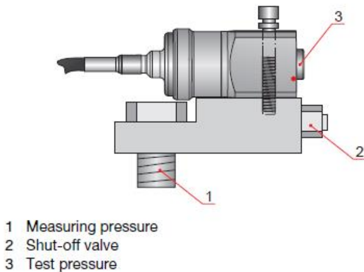
Slika 4. Testiranje senzora tlaka
