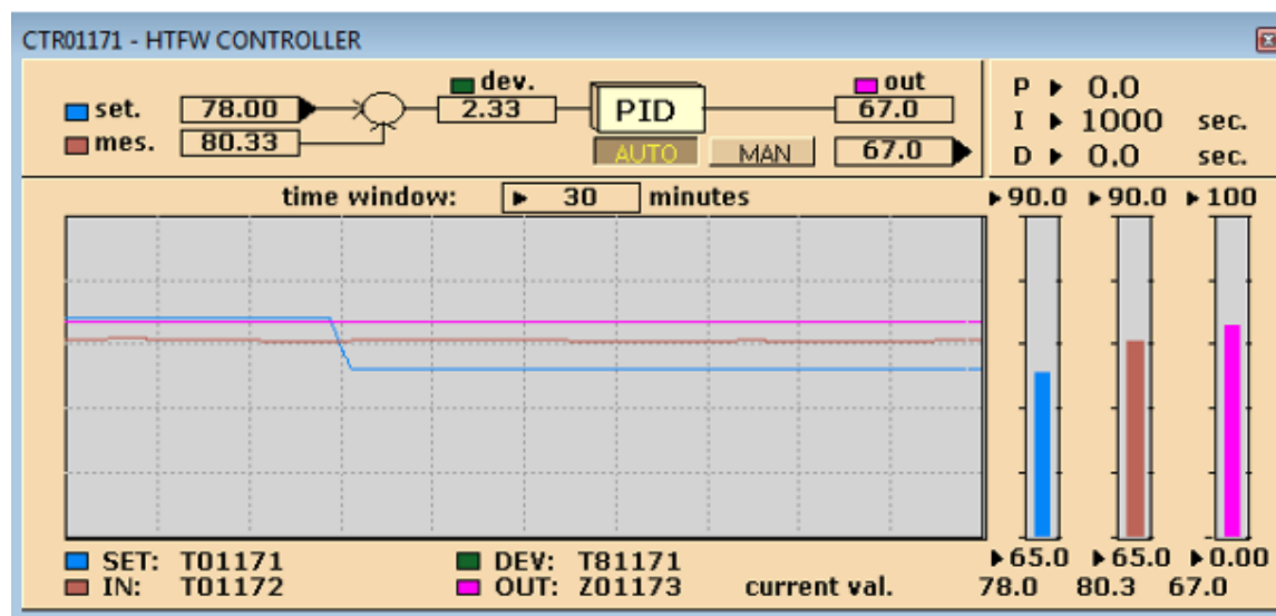
Slika 14. I regulator [3]
