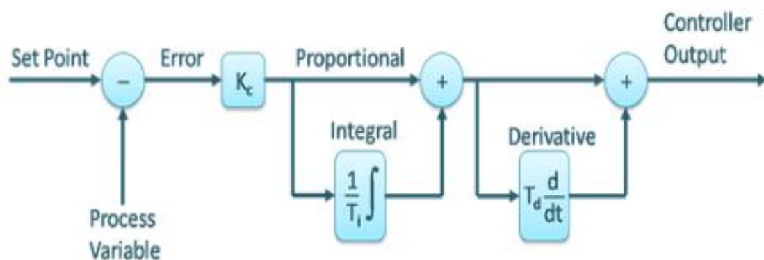
Slika 3. Interaktivni algoritam [5]
