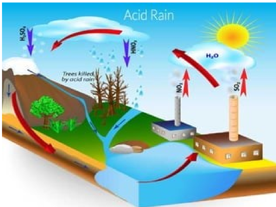
Slika 3. Nastanak kiselih kiša
