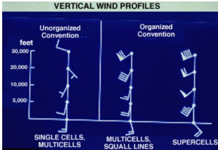
Slika 14. Smicanje vjetra
