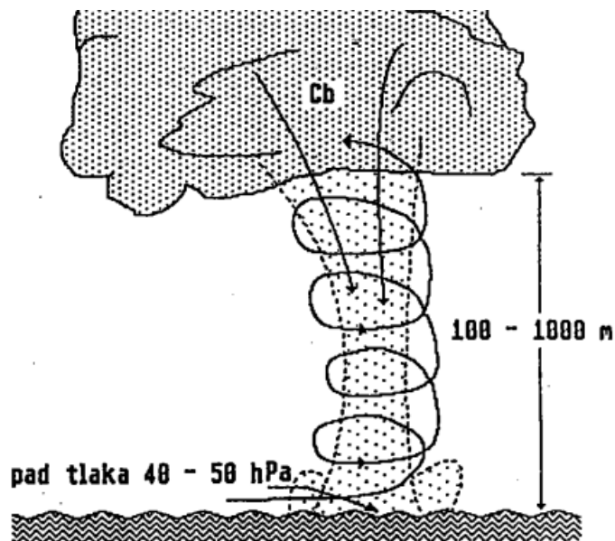
Slika 17. Pijavica
