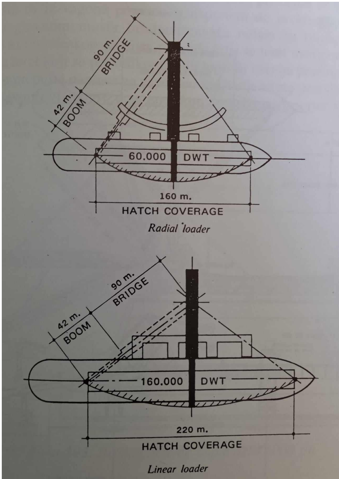
Slika4: Radijalni i linearni brodokrcavači za ukrcaj ugljena, željezne rude i boksita
