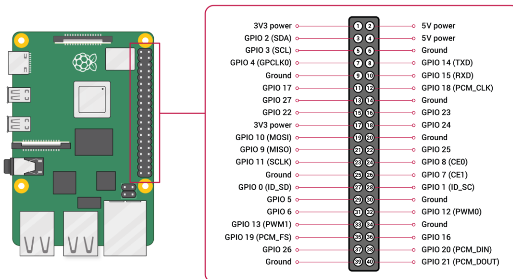
Slika 1 Raspored GPIO pinova na Raspberry Pi mikroročunalu Izvor: SparkFun
