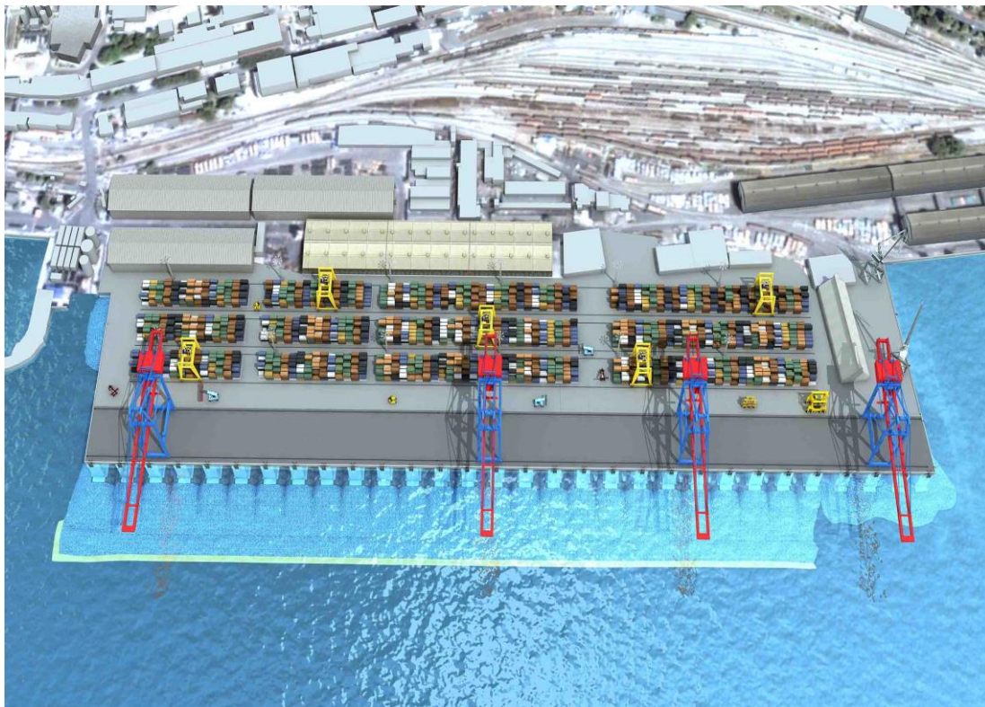
Slika 7: Kontejnerski terminal na Zagrebačkoj obali
