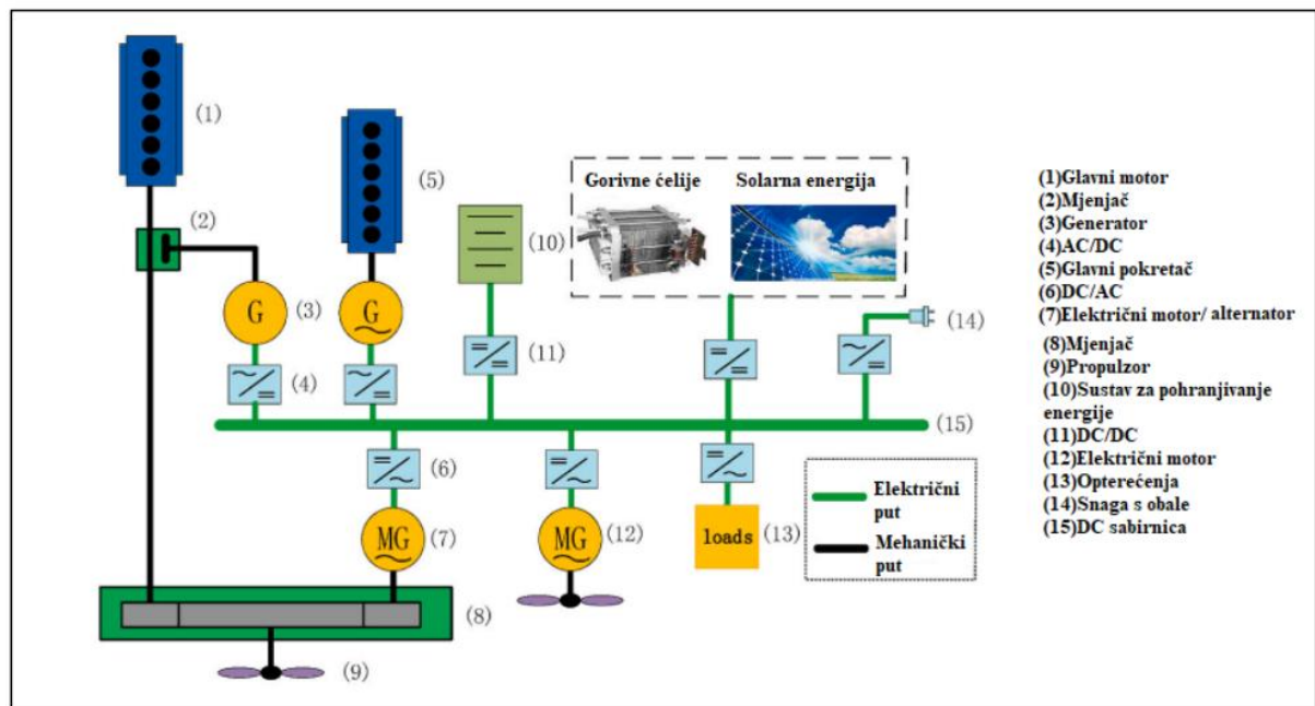
Slika 15. Shema hibridnog serijski-paralelnog elektroenergetskog sustava
