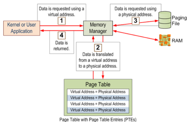
Slika 4: Upravitelj memorije
