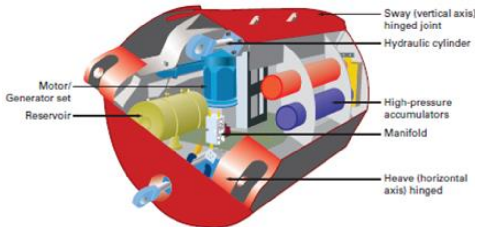
Slika 11: Prikaz presjeka hidrauličkog motora uređaja Pelamis
