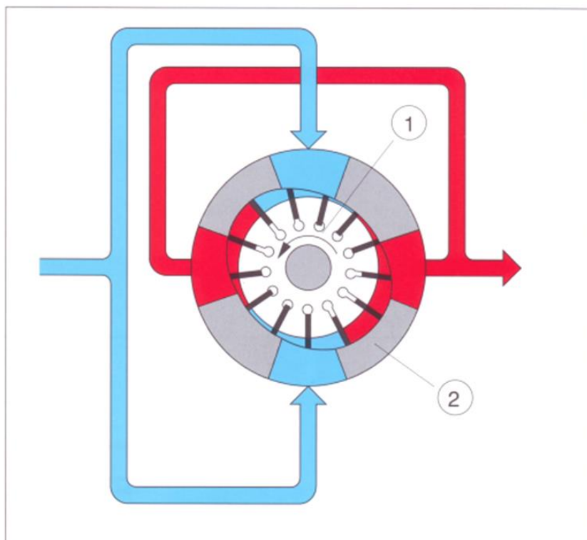
Slika 9. Krilna pumpa
