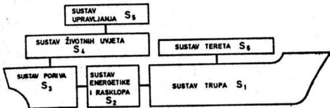
Slika 7. Brodski sustavi
