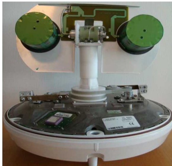
Slika 20. SAILOR 150 antenska jedinica
