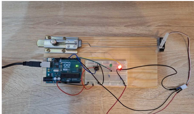
Slika 19. Kapacitivni senzor (fizička izvedba) – brava zatvorena Izvor: izradio autor (24.06.2024.)
