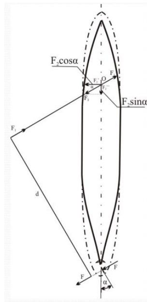
Slika 9 Djelovanje sile kormila
