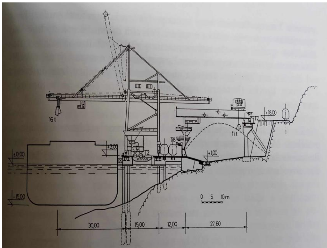
Slika 6. Prikaz brodoiskrcavača
