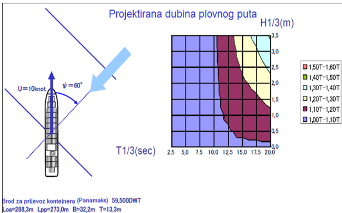
Slika 23: Prikaz određivanja potrebne dubine plovnog puta projektog tipa broda koristeći smjer, visinu i period signifikantnih valova
