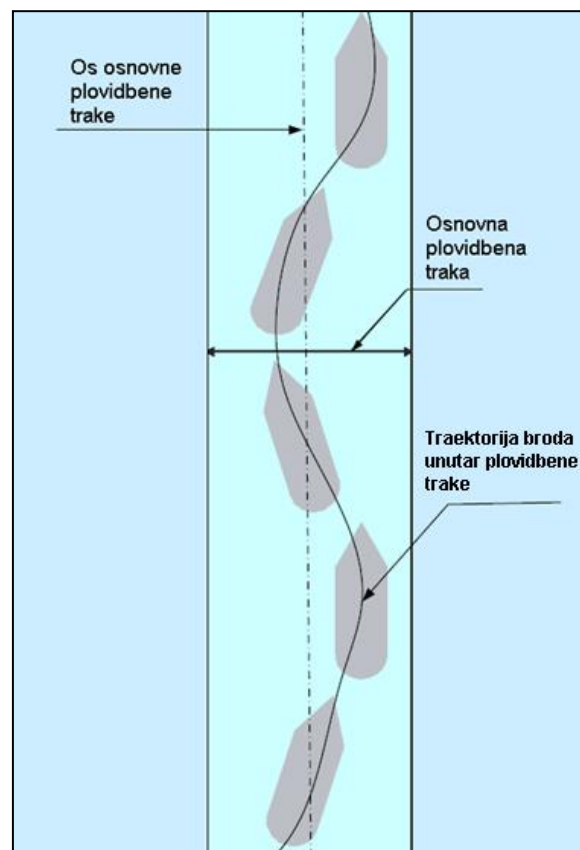
Slika 2: Prikaz utjecaja upravljivosti broda na širinu osnovne plovidbene trake
