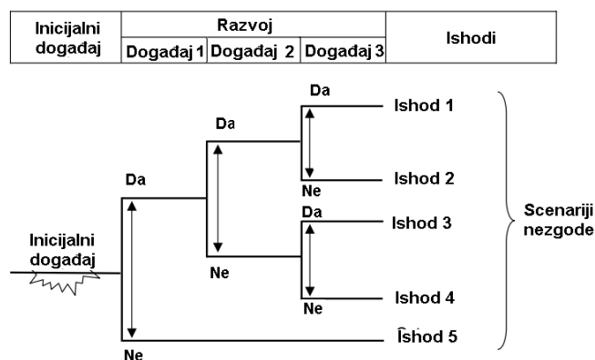
Slika 11: Koncept metode analize stabla događaja
